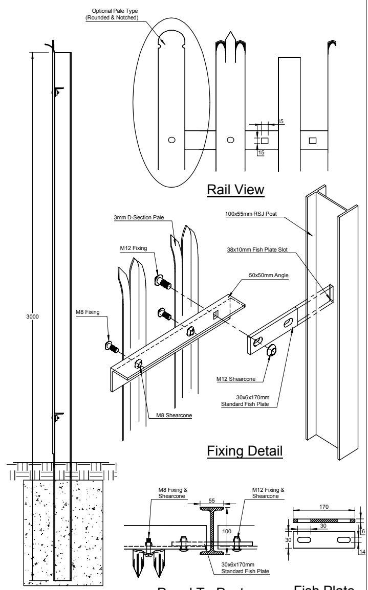
End Elevation
